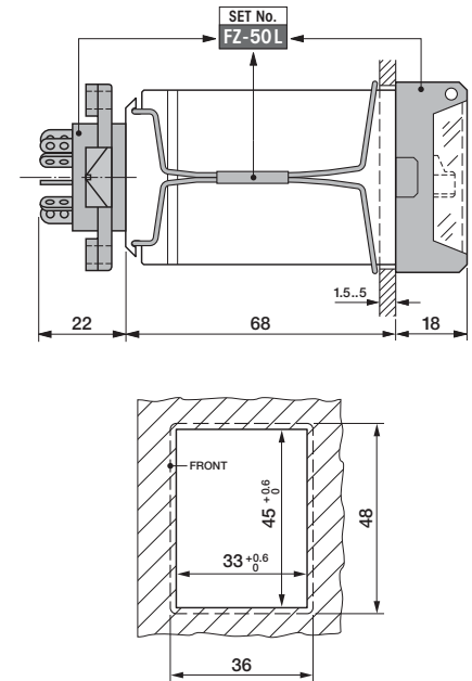
fig. 1. Dimensions (mm)
