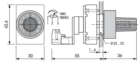
fig. 1. Dimensions (mm)
